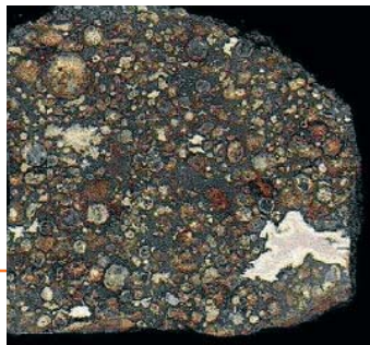
Meteorito de Allende. Un condrito ordinario donde se aprecian las condritas.
